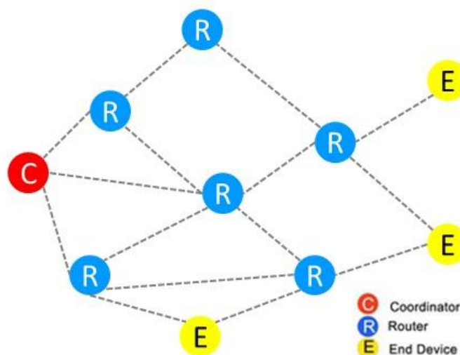
图 1-1 ZigBee 网络拓扑结构
