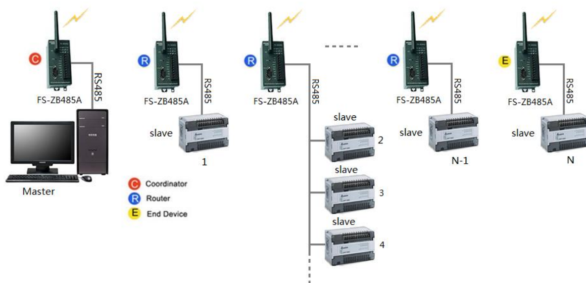
图5-2 ZigBee无线数采控制系统
