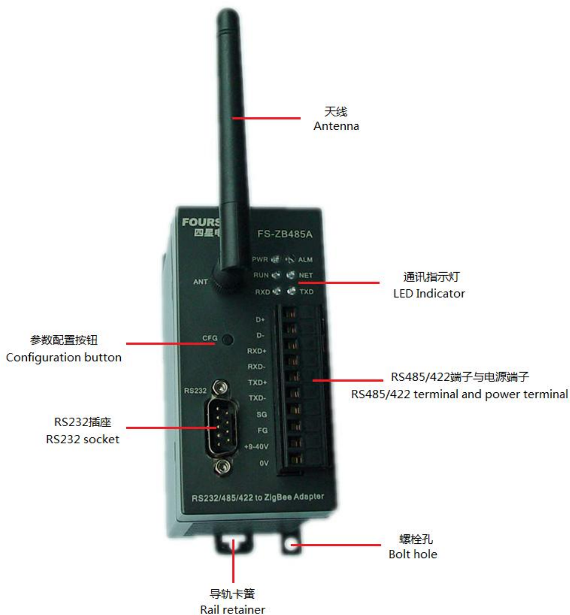
图3-1 FS-ZB485A适配器的外部结构及各部件说明
